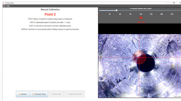
Capture d'écran du logiciel Perfect Zero mesurant différents points sur l'outil.
