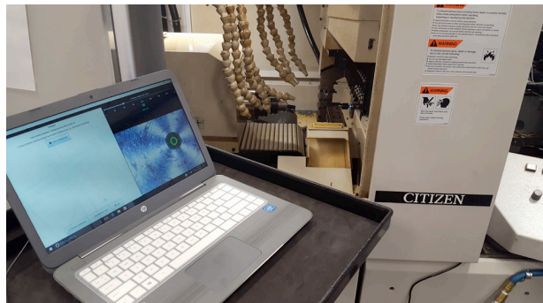
Perfect Zero réglant un outil coupant sur une CITIZEN à poupée mobile.
