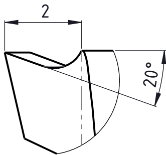
Y (10 : 1)
