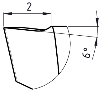
Y (10 : 1)
