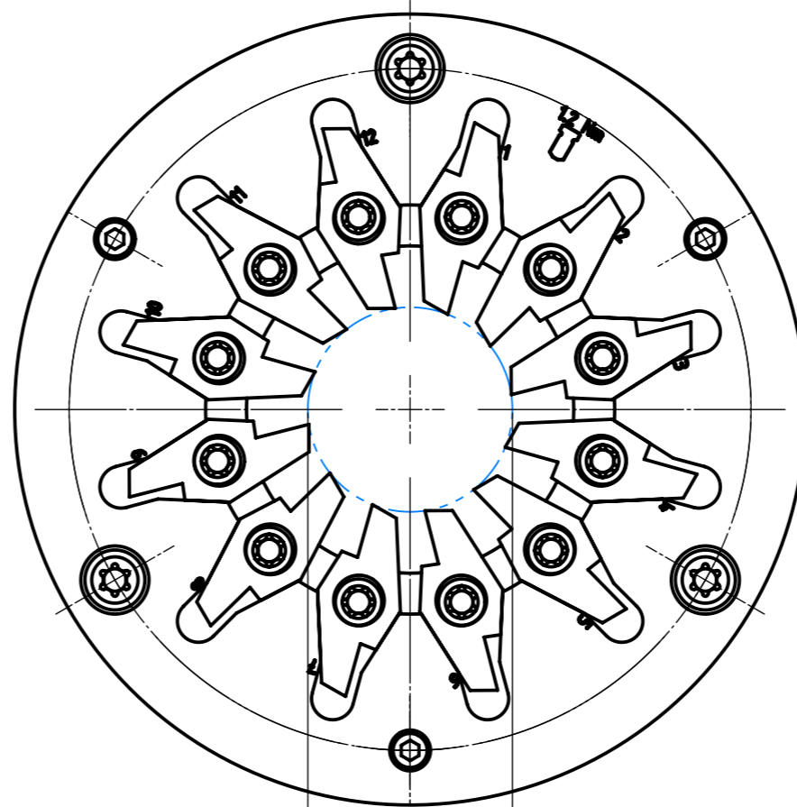
DF = Ø 15 Flugkreis Schneide Diamètre inscrit des couteaux Flight circle
