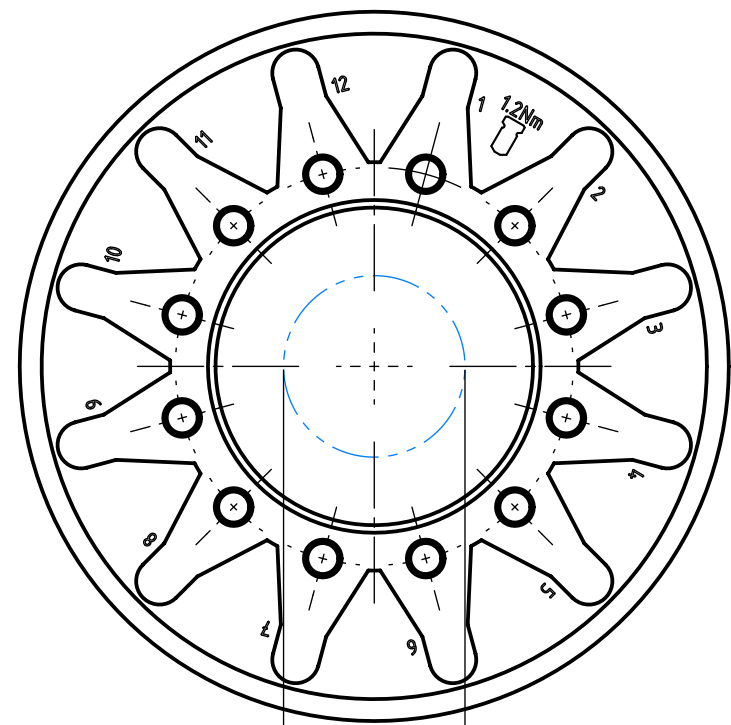
\varnothing 12 Flugkreis Schneide Diamètre inscrit des couteaux Flight circle
