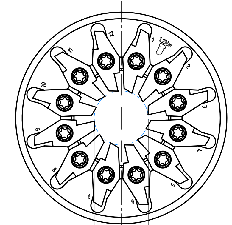
\varnothing 12 Flugkreis Schneide Diamètre inscrit des couteaux Flight circle
