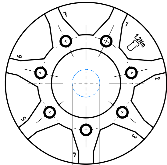
\varnothing 6 Flugkreis Schneide Diamètre inscrit des couteaux Flight circle
