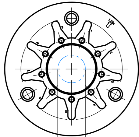
\phi 12 Flugkreis Schneide Diamètre inscrit des couteaux Flight circle
