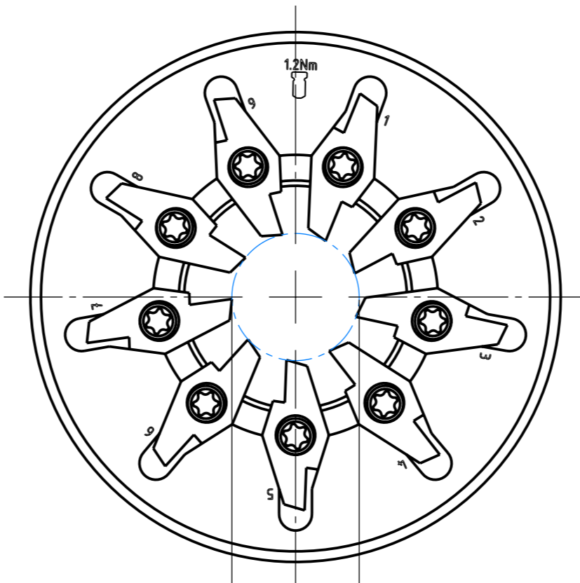
DF = Ø 12 Flugkreis Schneide Diamètre inscrit des couteaux Flight circle
